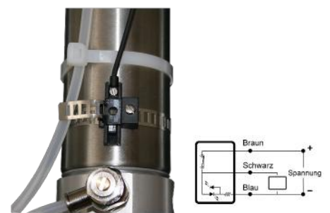
7002-0004 Füllstandsensor
